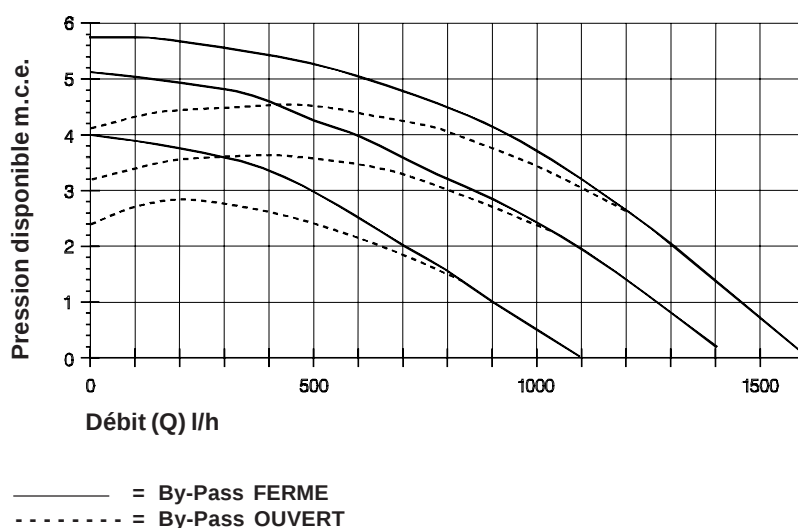
DIAGRAMME DEBIT/PRESSION DISPONIBLE POUR L'INSTALLATION
